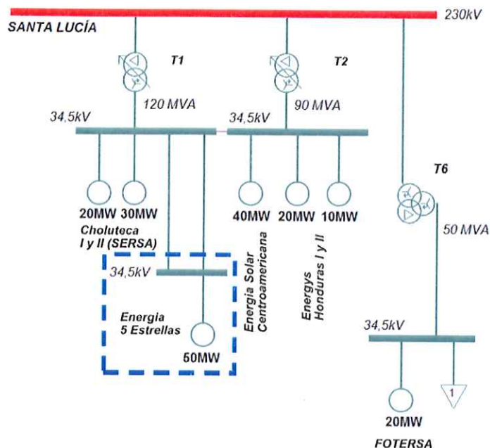
Figura 2: Esquema Unifilar de la subestación Santa Lucía donde se conecta el Proyecto.
